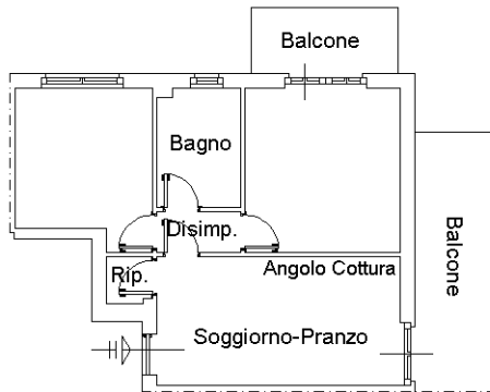
PIANO SECONDO CORPO "A" H=2.70
